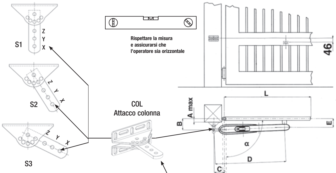
Misure da rispettare per una corretta installazione
