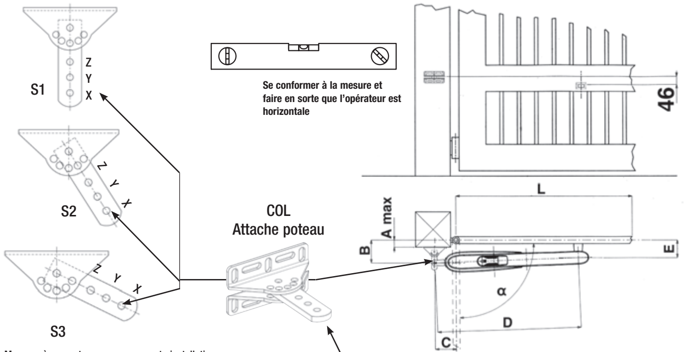
Mesures à respecter pour une correcte installation
