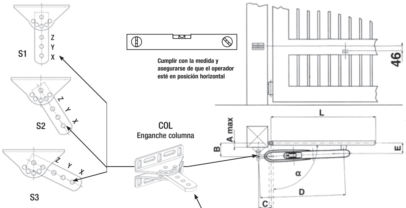
Medidas a respetar para una instalación correcta
