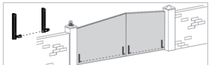
FOTOCÉLULAS SIN CABLES PARA REMPLAZAR A LA COSTA VERTIGO Wi-Fi 8 cód. ACG8042 - VERTIGO Wi-Fi 10
