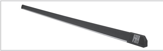
BARRE PALPEUSE MÉCANIQUE L = 2 m CERTIFIÉE EN 13849-2 (2008) - CATÉGORIE 3
