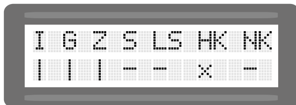
Impuls-, Gehtür- und ZU-Taster in Ordnung. STOPP-Taster und Lichtschranke nicht in Ordnung. Kontaktleiste (Hauptschließkante) unterbrochen. Kontaktleiste (Nebenschließkante) kurzgeschlossen.
