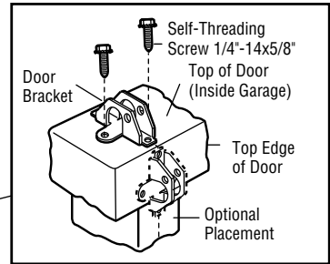
METAL DOOR
