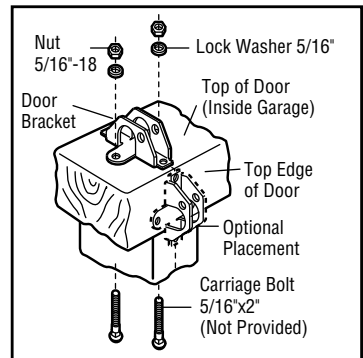
WOOD DOOR
