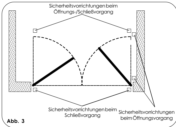
Anschluß eines Photozellenpaares beim Schließvorgang, eines Paares beim Öffnungsvorgang sowie eines Paares beim Öffnungs-/Schließvorgang (empfohlener Anschlußplan)
