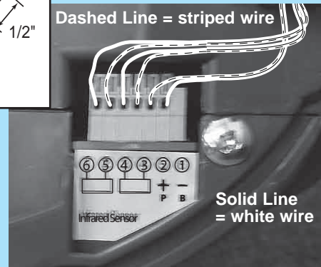
FIG. 4-8 Insert wires
