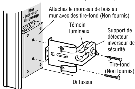
Figure 3 MONTAGE MURAL (CÔTÉ DROIT)
