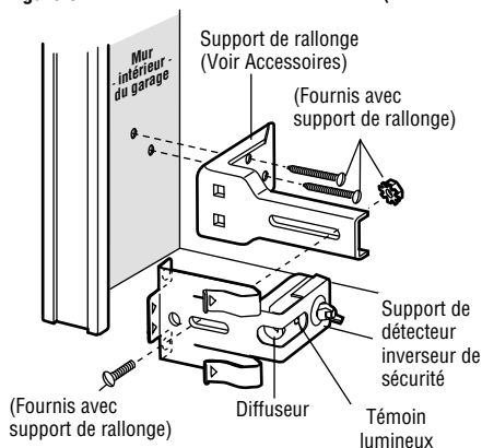
Figure 3 MONTAGE MURAL (CÔTÉ DROIT)
