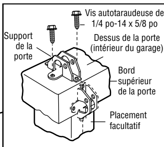
PORTE MÉTALLIQUE
