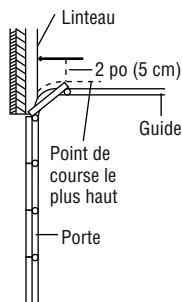
Porte articulée avec guide courbé
