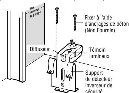
Figure 4 MONTAGE AU SOL (CÔTÉ DROIT)
