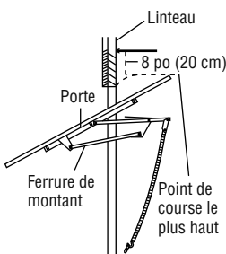
Porte rigide sans guides : ferrure de montant
