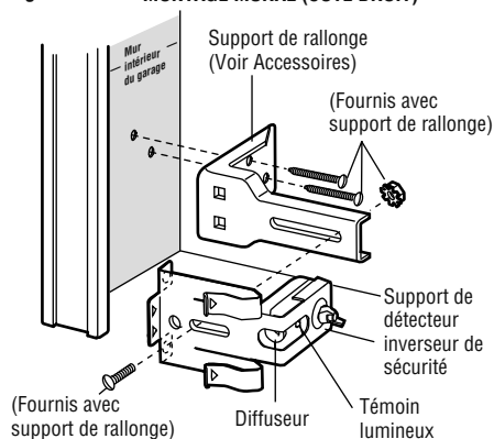
Figure 3 MONTAGE MURAL (CÔTÉ DROIT)
