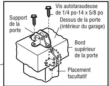
PORTE MÉTALLIQUE
